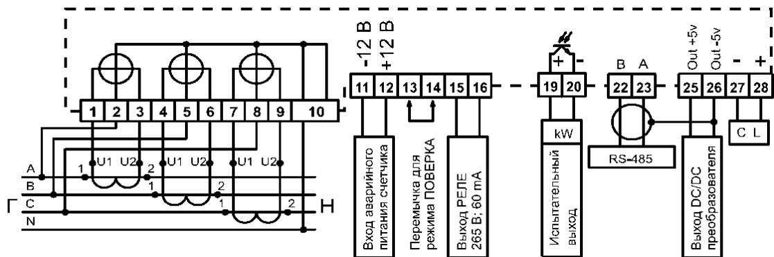
Рисунок 1 - Схемы подключения счетчика
