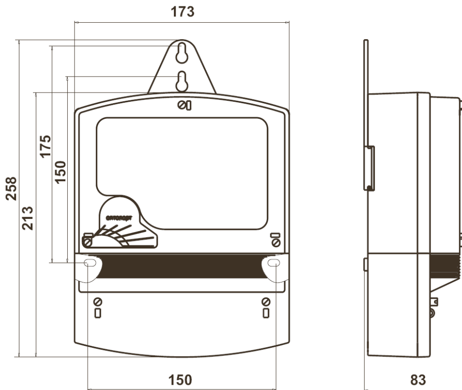
Рисунок 2 - Габаритные и установочные размеры счетчика
